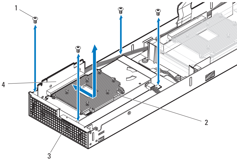
图 3-48. 卸下和安装正面 GPGPU 卡部件
