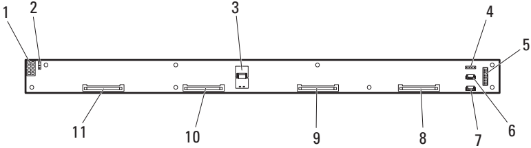
图 5-10. 3.5 英寸硬盘驱动器固定框架背板的正面视图
