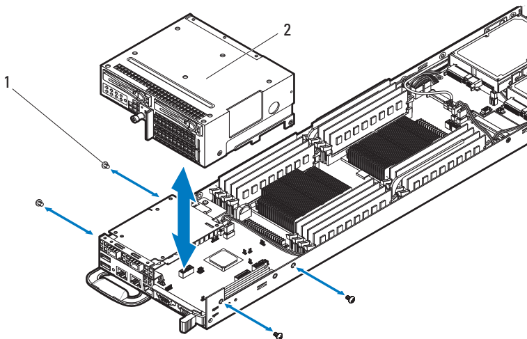
图 3-26. 卸下和安装正面机盖
