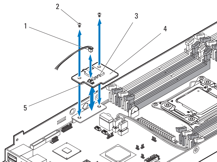
图 3-114. 卸下和安装 MicroSD 卡读取器
