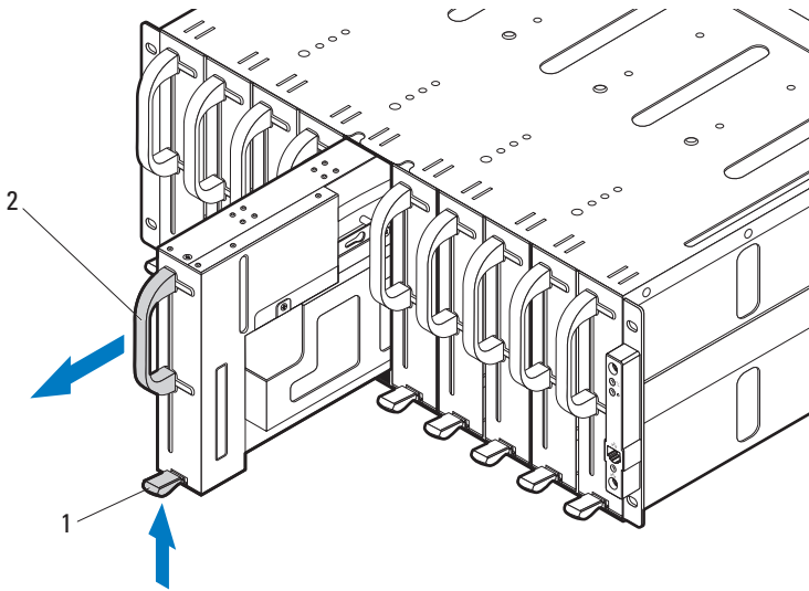
图 3-8. 卸下和安装单幅底座档片
