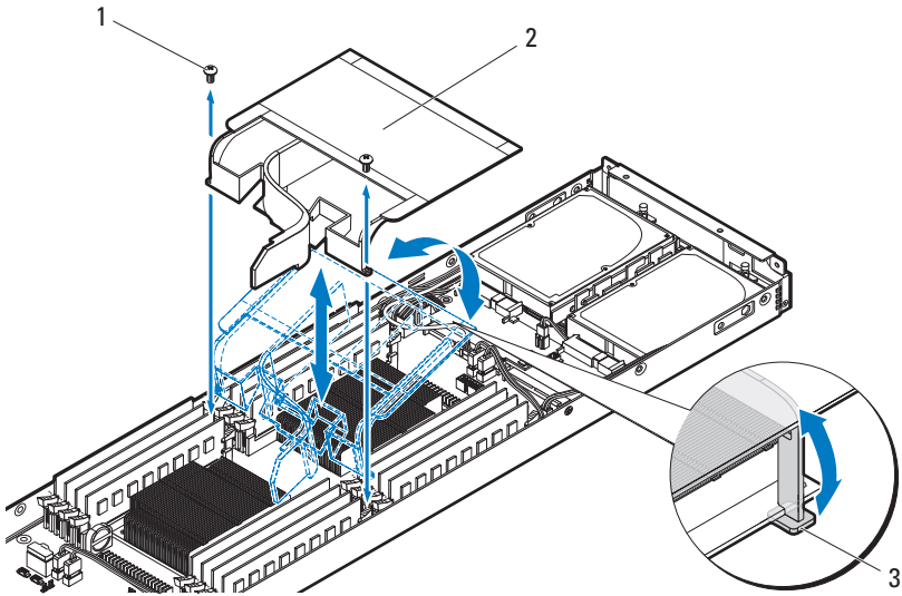
图 3-94. 卸下和安装冷却通风罩
