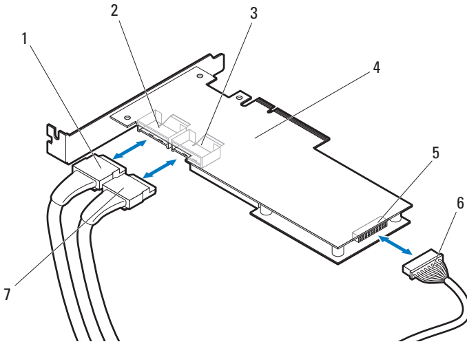
图 3-36. 断开和连接 MegaRAID SAS 9265-8i 卡电缆
