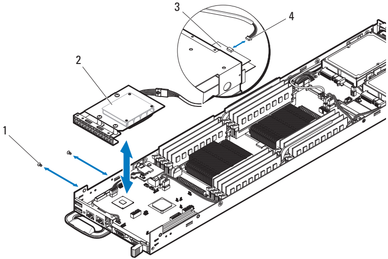
图 3-41. 卸下和安装 MegaRAID SAS 9285CV-8e RAID 电池
