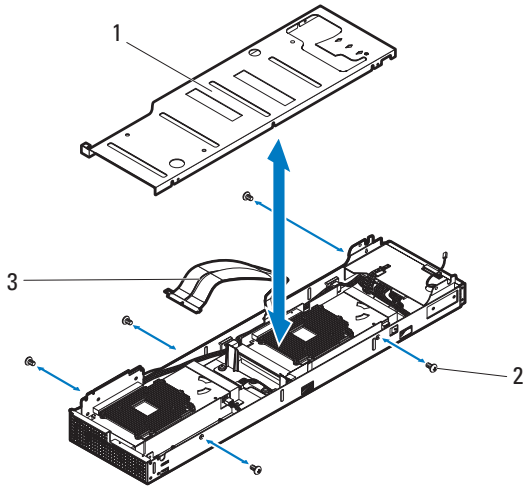
图 3-46. 卸下和安装顶盖
