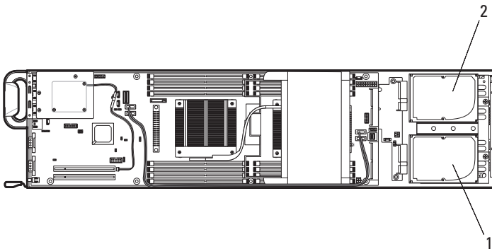
图 3-12. 内部 2.5 英寸硬盘驱动器
