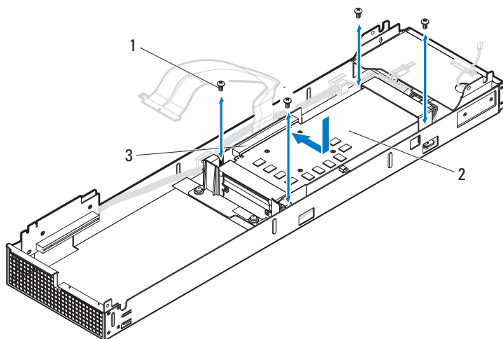
图 3-63. 卸下和安装背面 GPGPU 卡部件
