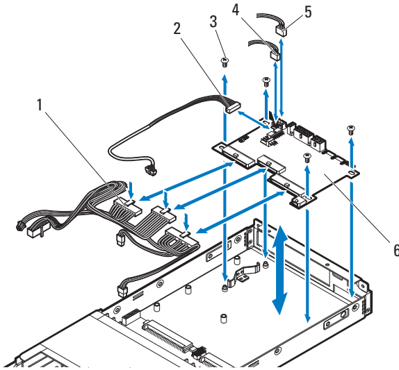
图 3-118. 卸下和安装节点配电板
