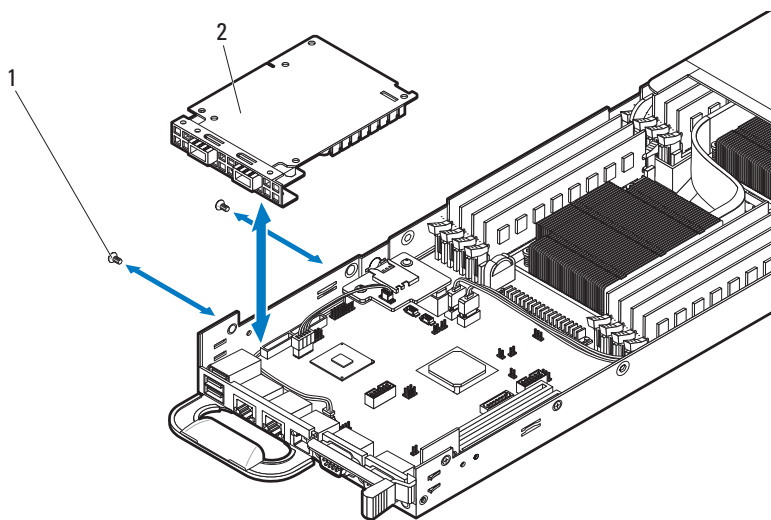
图 3-110. 卸下和安装 10 GbE 夹层卡部件
