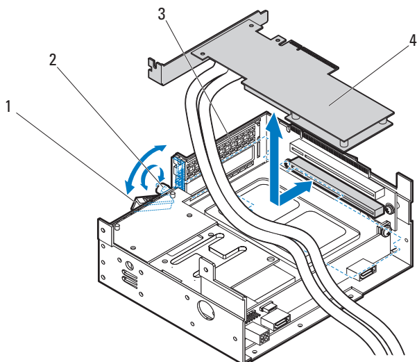
图 3-35. 卸下和安装 MegaRAID SAS 9265-8i 卡
