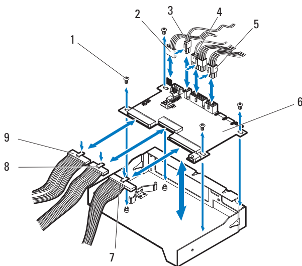
图 3-120. 卸下和安装节点配电板
