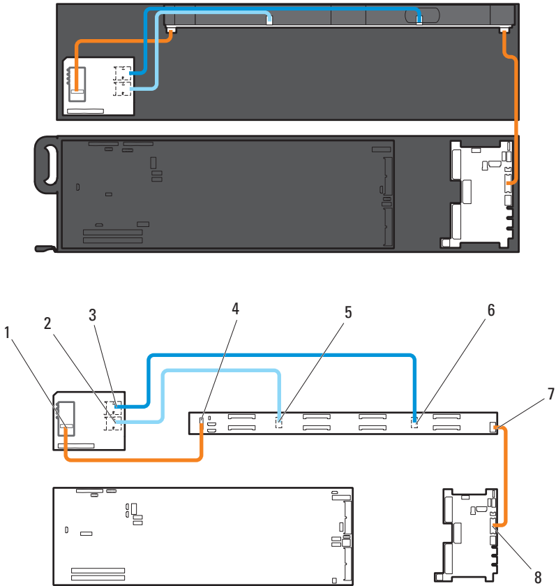
图 3-105. SAS 夹层卡的电缆布线 (2.5 英寸硬盘驱动器背板)
