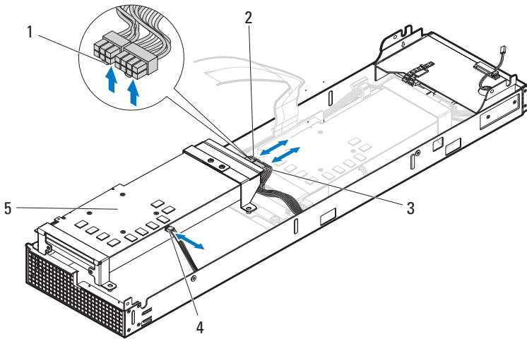
图 3-59. 卸下和安装正面 GPGPU 卡电缆
