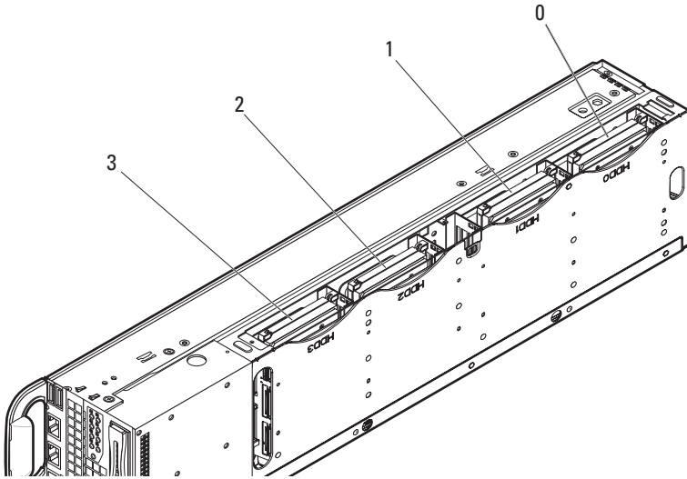
图 3-12. 内部 2.5 英寸硬盘驱动器
