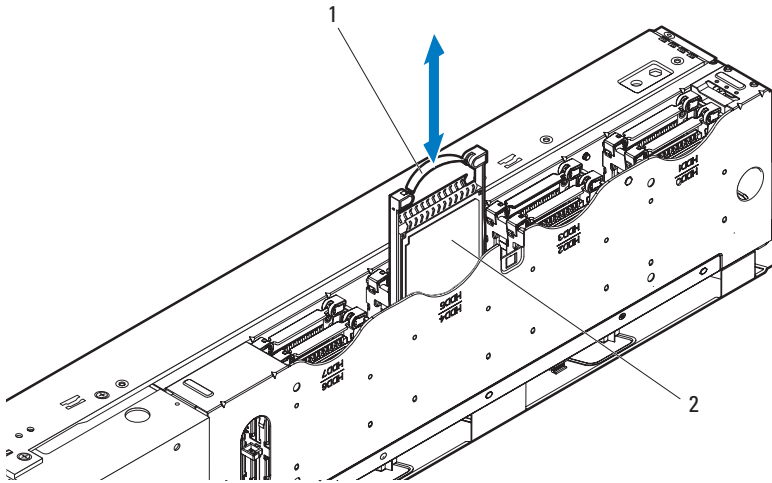
图 3-17. 卸下位于底座盖中的硬盘驱动器托盘，再将其安装
