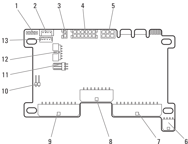
图 5-16. 节点配电板连接器
