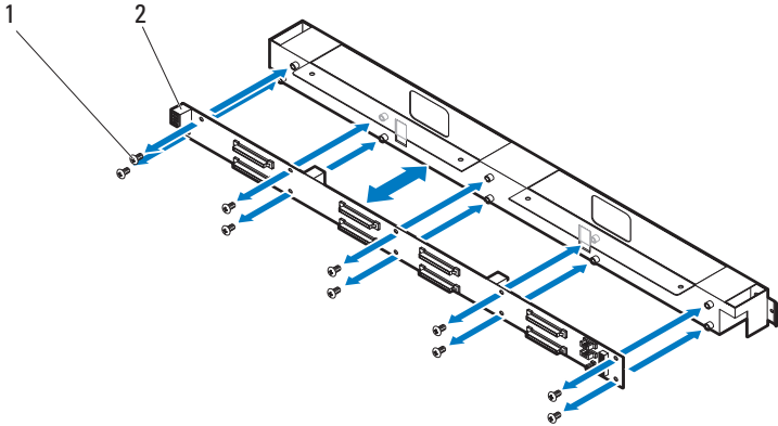
图 3-91. 卸下和安装 2.5 英寸硬盘驱动器背板
