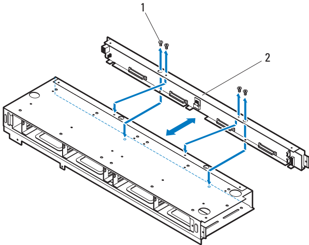
图 3-92. 卸下和安装 3.5 英寸硬盘驱动器固定框架背板部件
