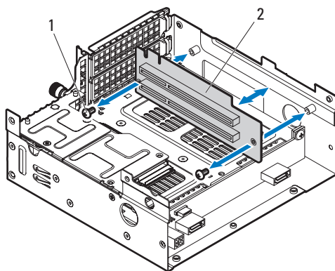
图 3-45. 卸下和安装扩展卡提升板
