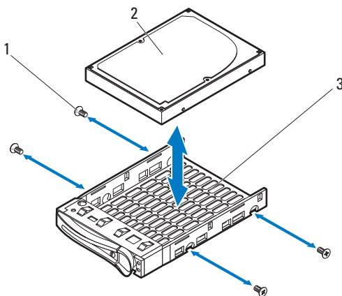
图 3-15. 从硬盘驱动器托盘中卸下硬盘驱动器，然后再安装
