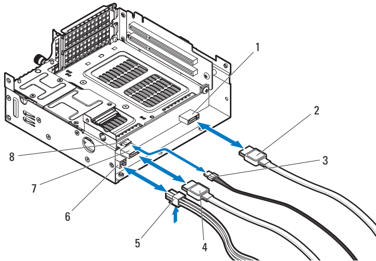
图 3-30. 断开和连接热插拔硬盘驱动器背板电缆
