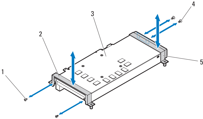
图 3-71. 卸下和安装正面 NVIDIA Tesla K20 GPGPU 卡
