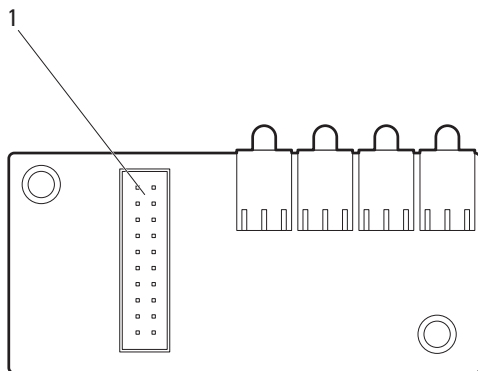
图 5-12. 硬盘驱动器 LED 板连接器
