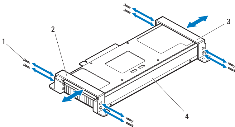
图 3-85. 卸下和安装背面 Xeon Phi 5110P/7120P 卡
