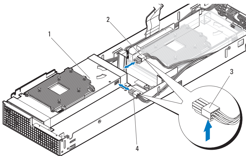
图 3-49. 卸下和安装正面 GPGPU 卡电缆
