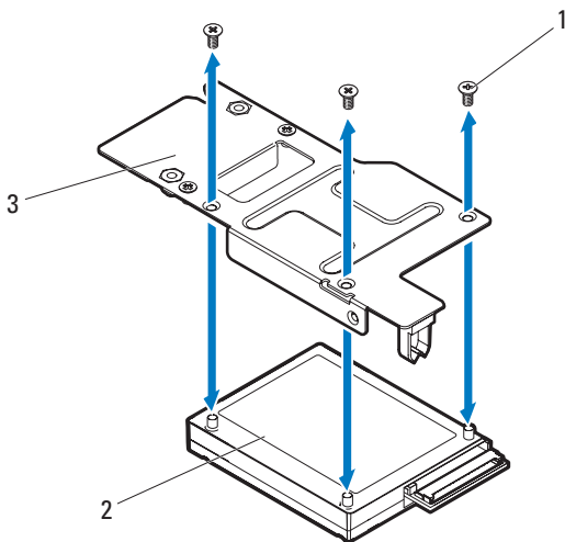
图 3-40. 卸下和安装 MegaRAID SAS 9265-8i RAID 电池
