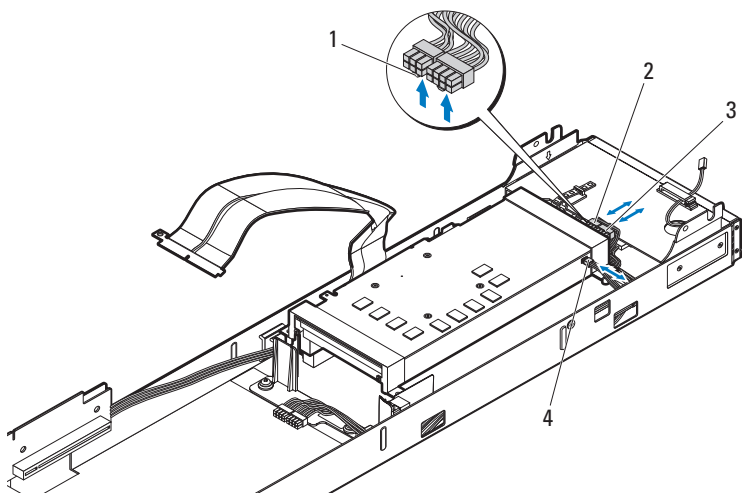
图 3-74. 卸下和安装背面 GPGPU 卡电缆
