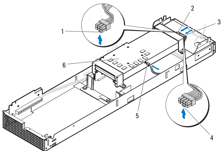
图 3-64. 卸下和安装正面 GPGPU 卡电缆
