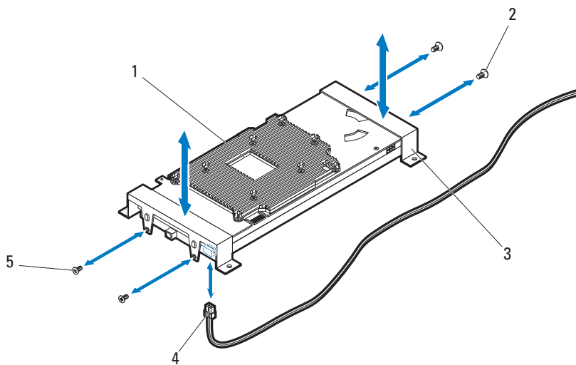
图 3-55. 卸下和安装背面 NVIDIA Tesla M2090 GPGPU 卡
