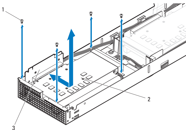
图 3-68. 卸下和安装正面 GPGPU 卡部件
