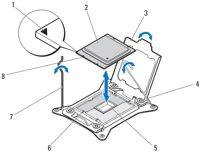
图 3-98. 卸下和安装处理器
