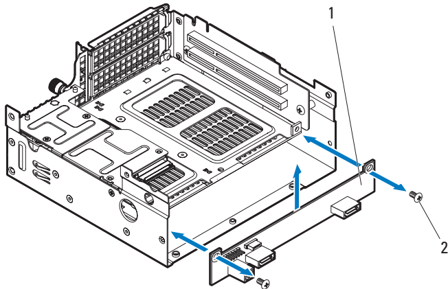
图 3-32. 卸下和安装 2.5 英寸热插拔硬盘驱动器背板
