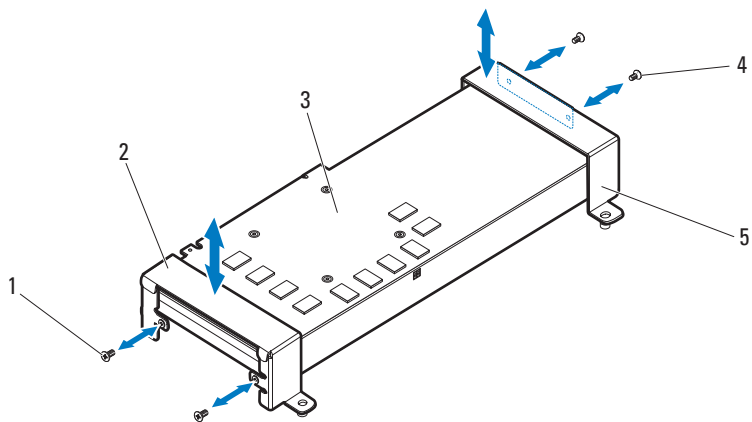
图 3-65. 卸下和安装背面 NVIDIA Tesla K10 GPGPU 卡
