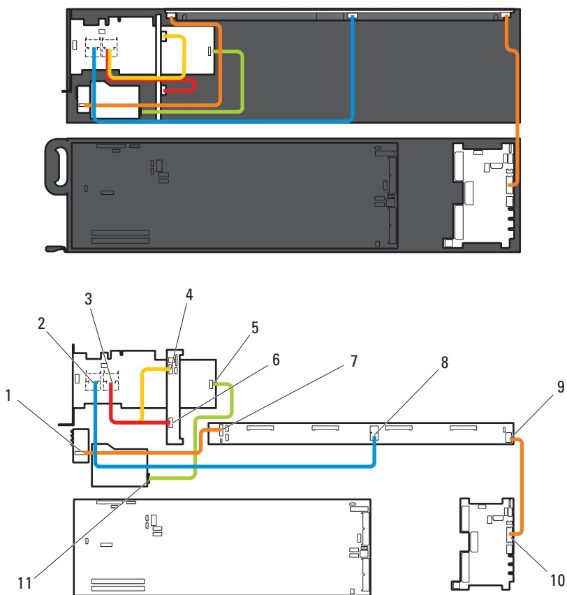
图 3-38. MegaRAID SAS 9265-8i 卡（3.5 英寸硬盘驱动器背板）的电缆布线
