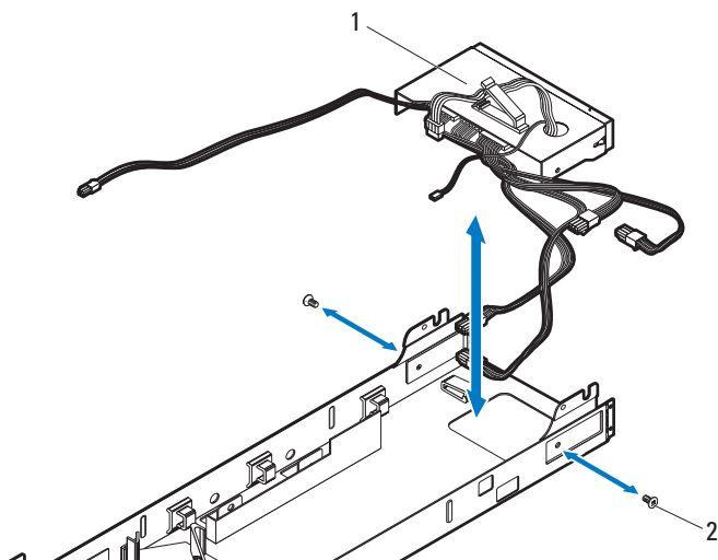
图 3-119. 卸下和安装节点配电板
