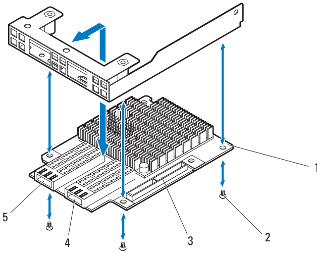
图 3-109. 卸下和安装 Infiniband 夹层卡
