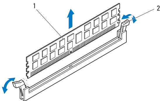
图 3-100. 卸下内存模块
