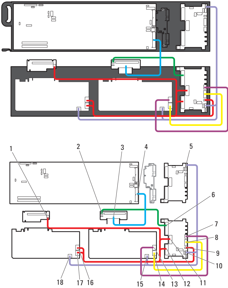
图 3-70. 正面和背面 NVIDIA Tesla K20 GPGPU 卡部件的电缆布线
