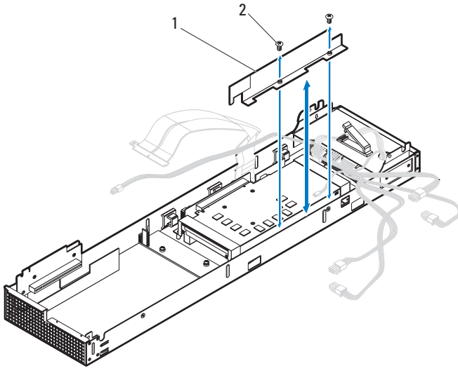
图 3-72. 卸下和安装空气导流板
