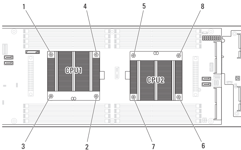
图 3-95. 散热器螺钉拧松顺序
