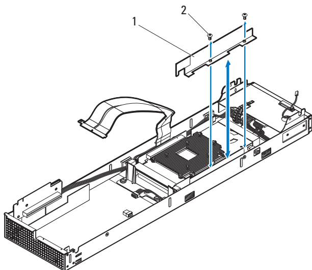
图 3-52. 卸下和安装空气导流板
