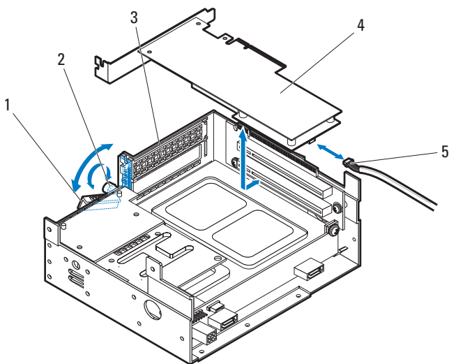
图 3-39. 卸下和安装 MegaRAID SAS 9285CV-8e 卡
