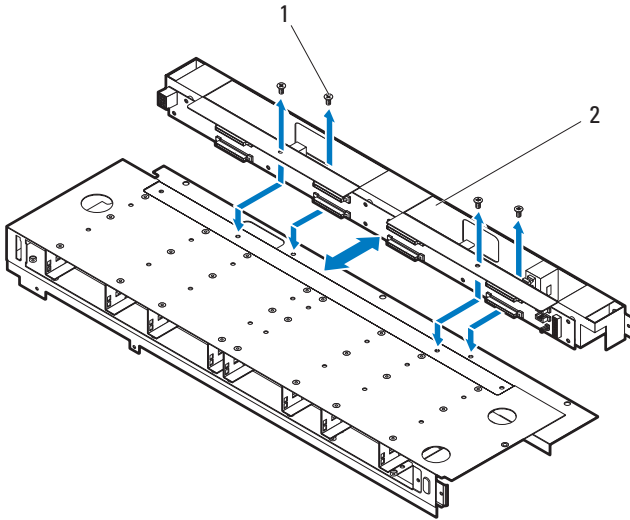
图 3-90. 卸下和安装 2.5 英寸硬盘驱动器固定框架背板部件
