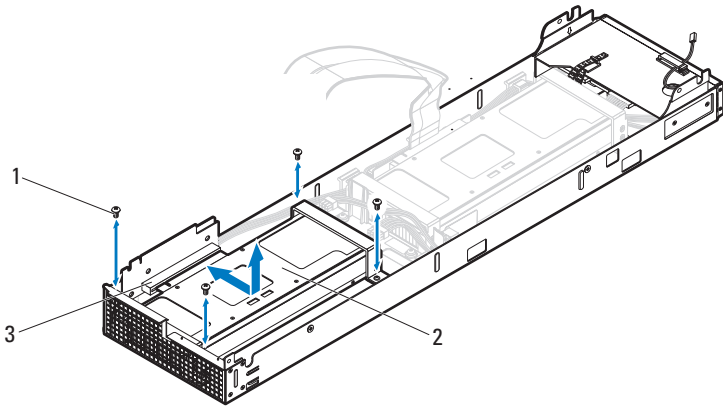
图 3-78. 卸下和安装正面 Xeon Phi 5110P/7120P 卡部件
