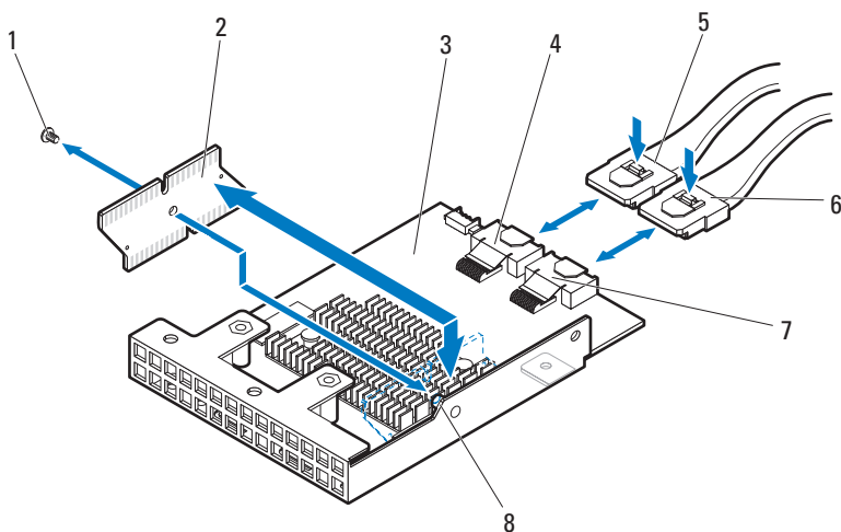
图 3-103. 卸下和安装夹层卡桥接板
