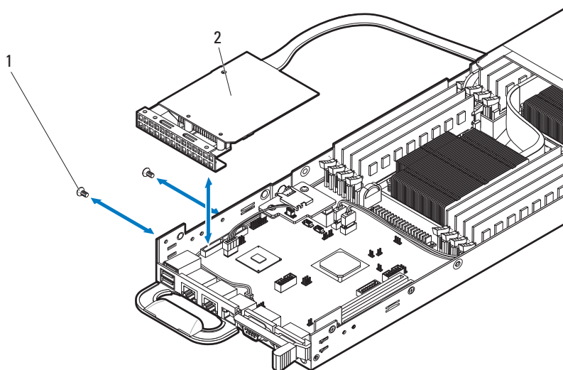
图 3-102. 卸下和安装 SAS 夹层卡部件
