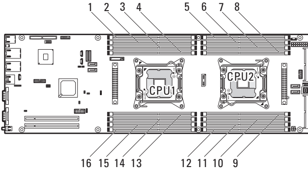
图 3-99. 内存插槽位置
