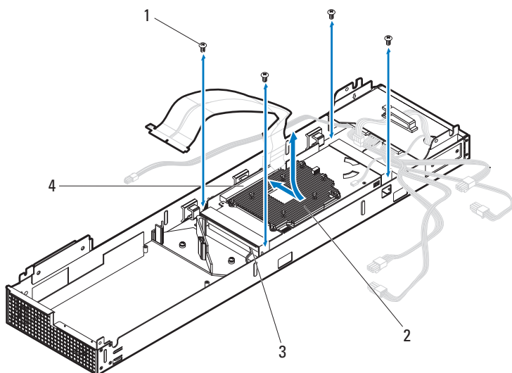
图 3-53. 卸下和安装背面 GPGPU 卡部件
