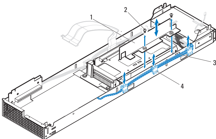
图 3-82. 卸下和安装空气导流板
