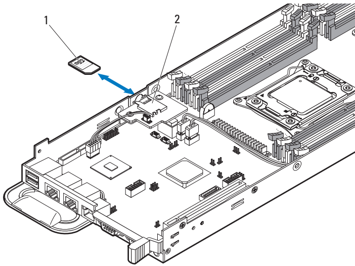
图 3-113. 卸下和安装 MicroSD 卡
