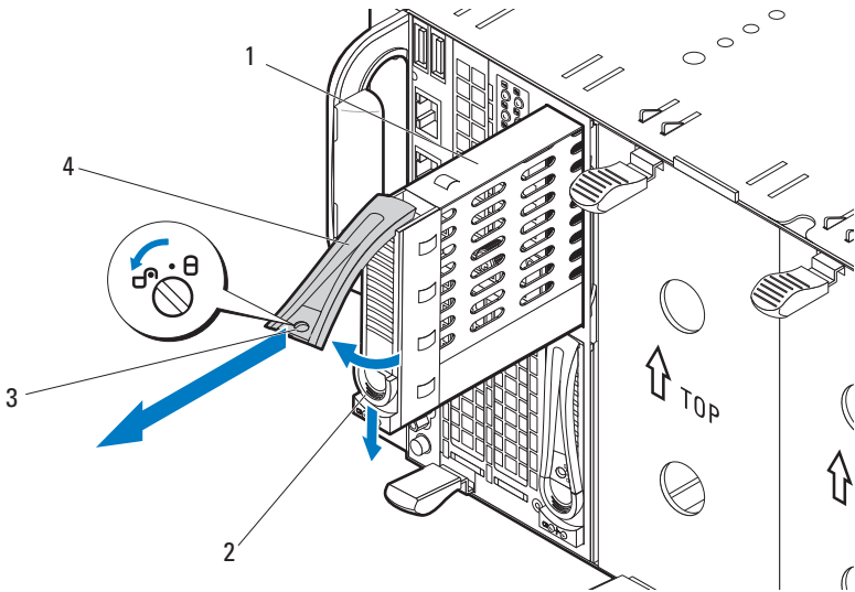
图 3-13. 卸下和安装硬盘驱动器挡片
