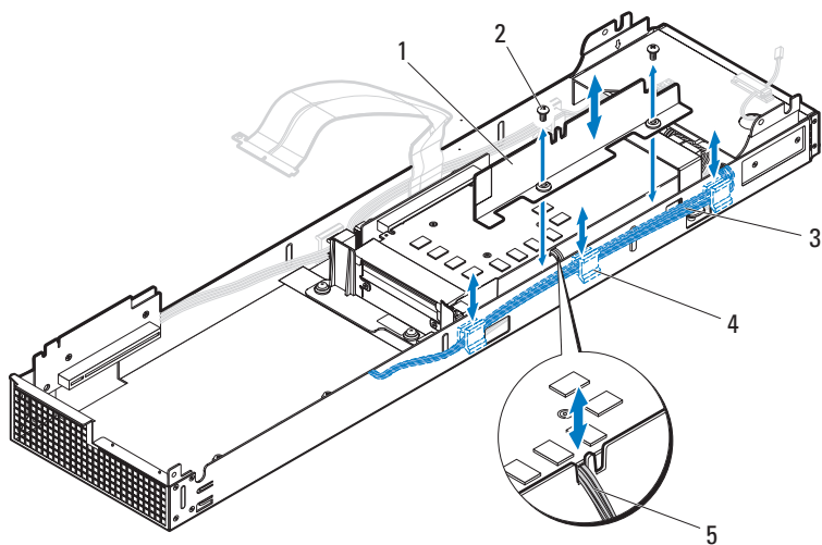
图 3-62. 卸下和安装空气导流板
