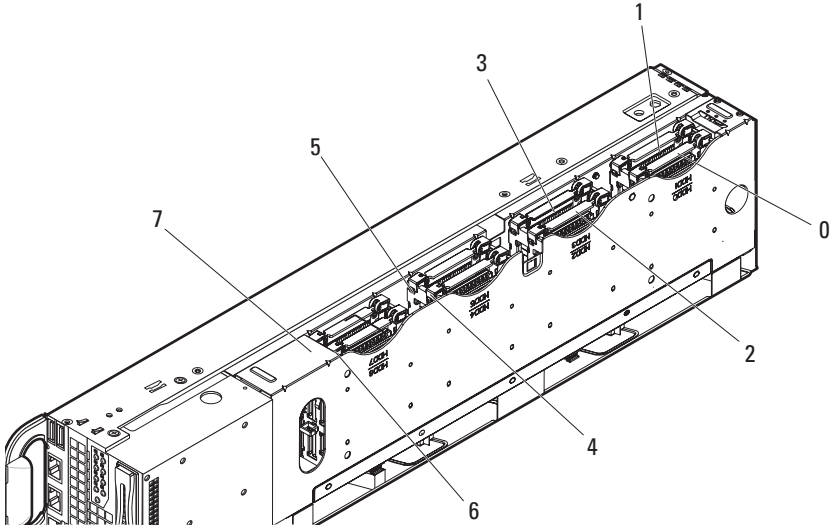
图 3-10. 硬盘驱动器固定框架硬盘驱动器 — 2.5 英寸 (8 驱动器托架) 硬盘驱动器
