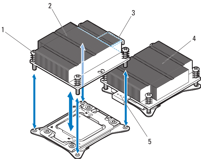
图 3-96. 卸下和安装散热器
