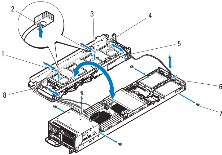
图 3-24. 从带添加式插卡的底座卸下和安装 8 驱动器托架背面盖
