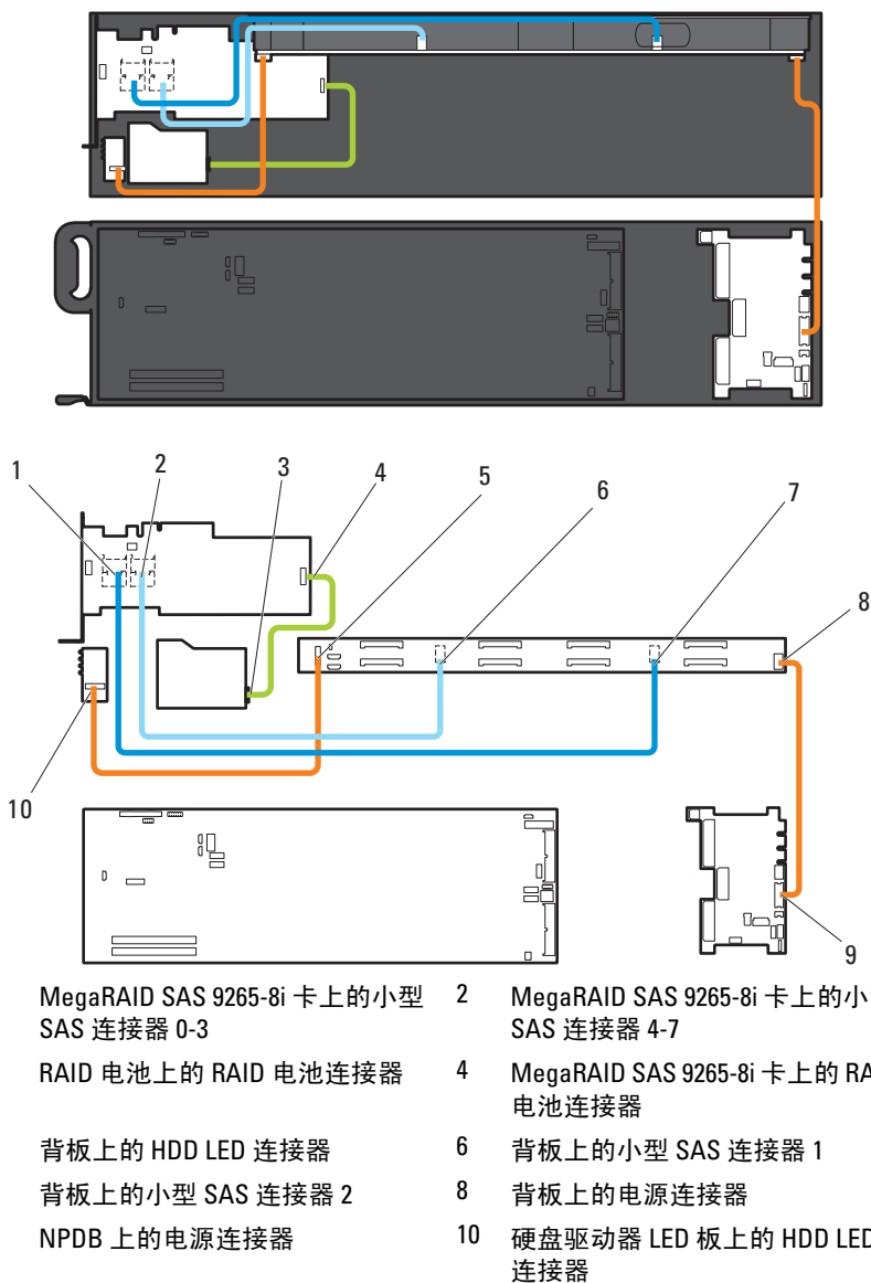
图 3-37. MegaRAID SAS 9265-8i 卡（2.5 英寸硬盘驱动器背板）的电缆布线
