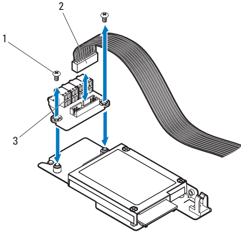
图 3-34. 卸下和安装硬盘驱动器 LED 板
