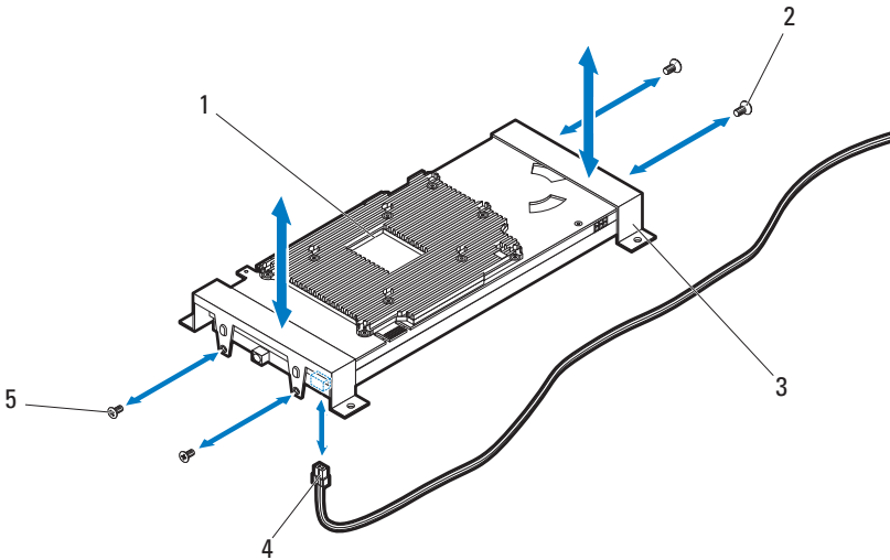
图 3-51. 卸下和安装正面 NVIDIA Tesla M2090 GPGPU 卡
