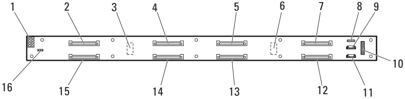
图 5-9. 2.5 英寸硬盘驱动器固定框架背板
