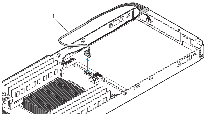
图 3-124. 卸下和安装系统板控制电缆
