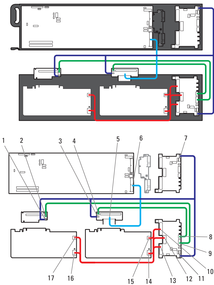
图 3-80. 正面和背面 Xeon Phi 5110P/7120P 卡部件的电缆布线
