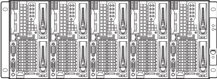
图 3-5. PowerEdge C8220X 4 底座 SKU
