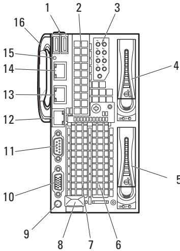
图 1-1. 底座正面功能部件 — C8220X 双幅计算底座，带前部访问的 2.5 英寸热插拔硬盘驱动器
