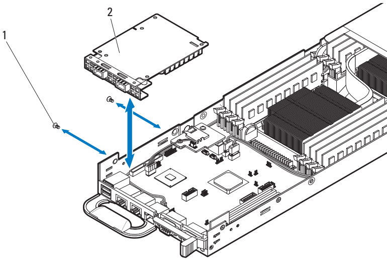
图 3-107. 卸下和安装 Infiniband 夹层卡部件
