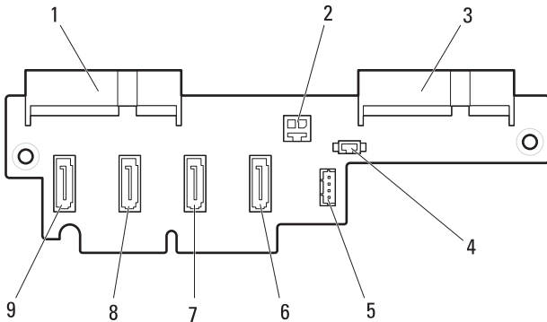
图 5-13. 插入器延长器 V1.0 连接器
