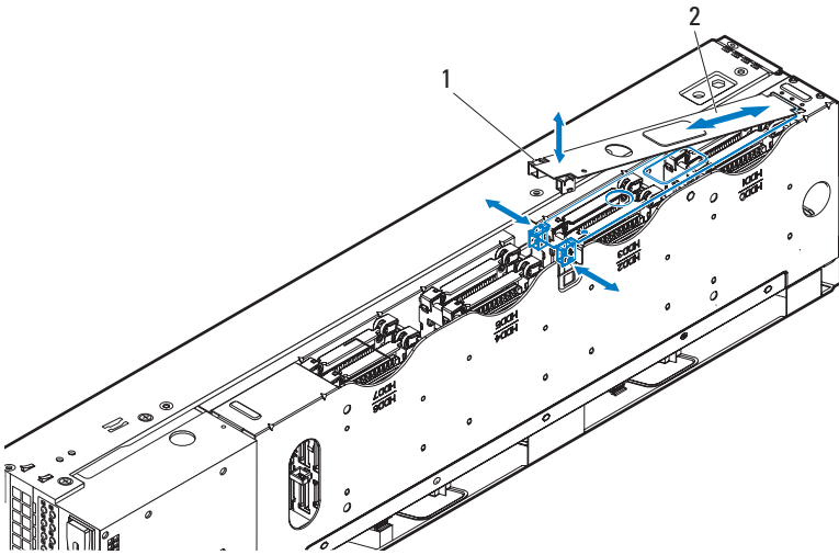
图 3-16. 打开并关闭驱动器托架盖
