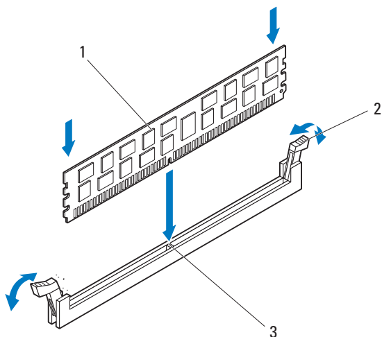
图 3-101. 安装内存模块
