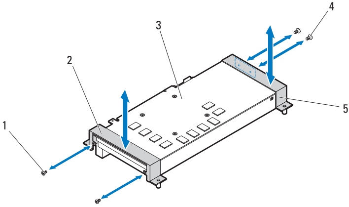
图 3-75. 卸下和安装背面 NVIDIA Tesla K20 GPGPU 卡
