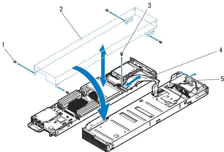
图 3-28. 卸下和安装底座盖
