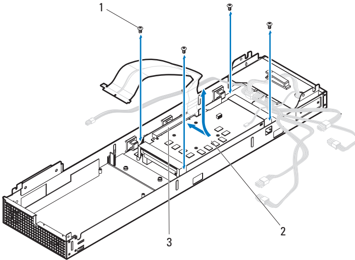
图 3-73. 卸下和安装背面 GPGPU 卡部件
