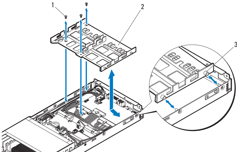
图 3-21. 卸下和安装硬盘驱动器托架
