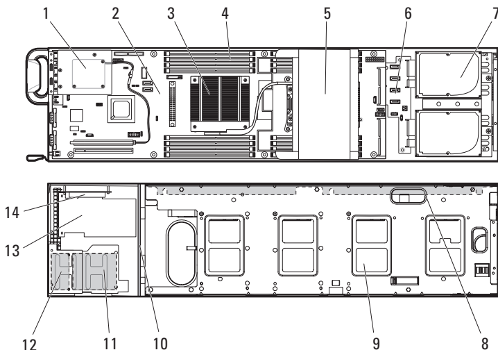
图 3-1. 带 3.5 英寸（4 驱动器托架）硬盘驱动器的 C8220X 的内部组件
