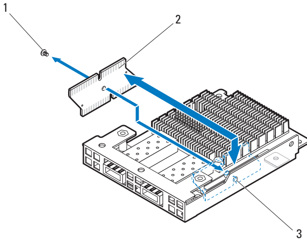
图 3-111. 卸下和安装夹层卡桥接板
