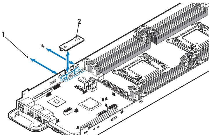
图 3-115. 卸下和安装 MicroSD 卡读取器支撑架
