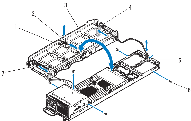
图 3-25. 从带添加式插卡的底座卸下和安装 4 驱动器托架背面盖
