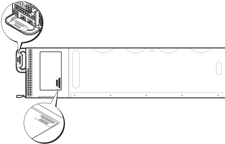
图 1-11. 带有 3.5 英寸 (4 驱动器托架) 硬盘驱动器的 C8220X 的服务标签位置
