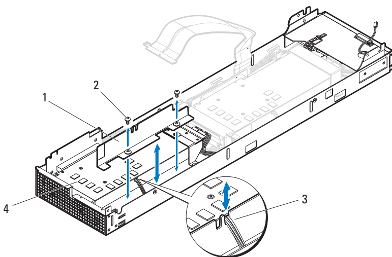
图 3-57. 卸下和安装空气导流板
