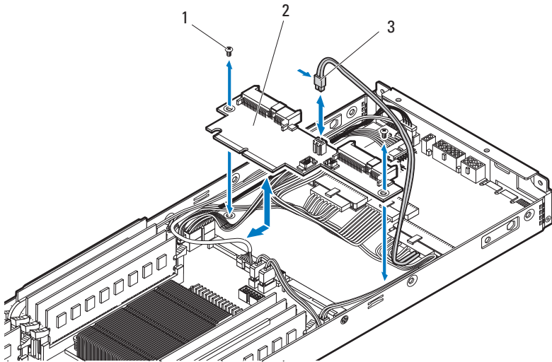
图 3-116. 卸下和安装插入器延长器
