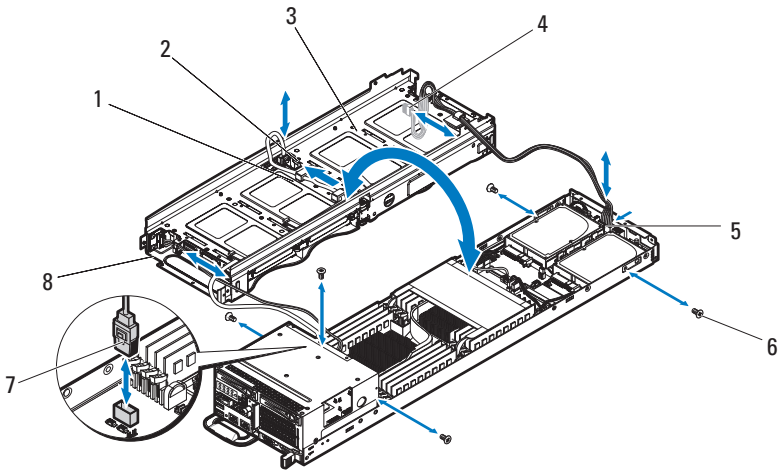
图 3-23. 从带添加式插卡的底座卸下和安装 4 驱动器托架背面盖
