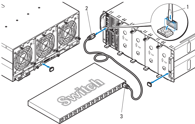
图 1-5. 非中央独立模式
