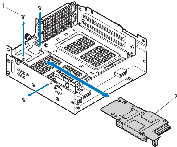
图 3-33. 卸下和安装硬盘驱动器 LED 板部件
