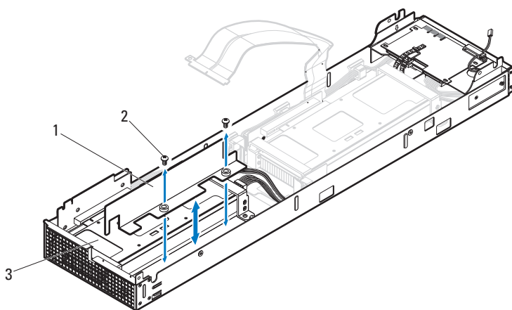
图 3-77. 卸下和安装空气导流板
