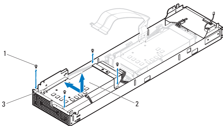
图 3-58. 卸下和安装正面 GPGPU 卡部件
