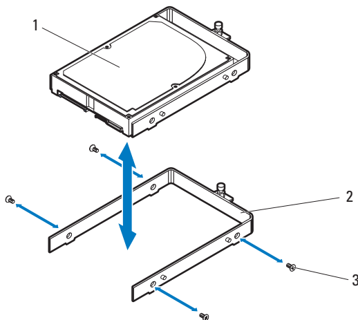
图 3-20. 从硬盘驱动器托盘中卸下硬盘驱动器，然后再安装
