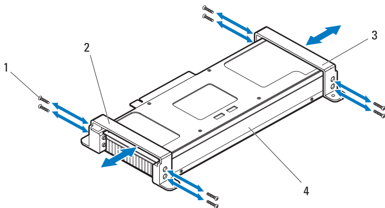
图 3-81. 卸下和安装正面 Xeon Phi 5110P/7120P 卡
