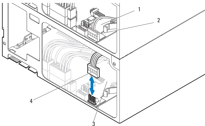
图 3-29. 连接紧急节流电缆
