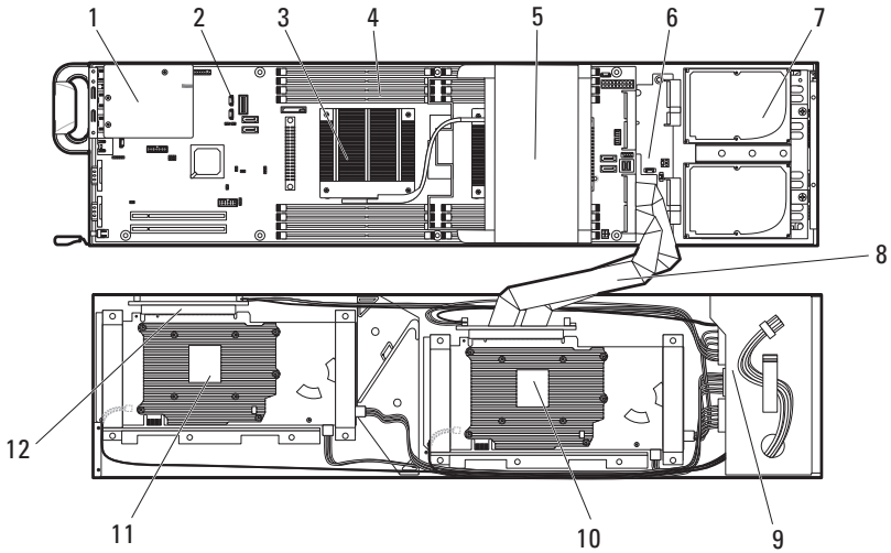
图 3-3. 带 GPGPU/Xeon Phi 卡的 C8220X 的内部组件
