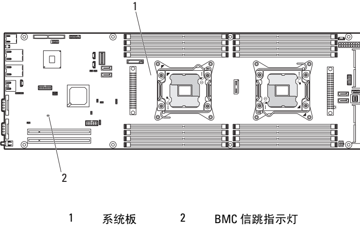
图 1-10. BMC 信跳指示灯
