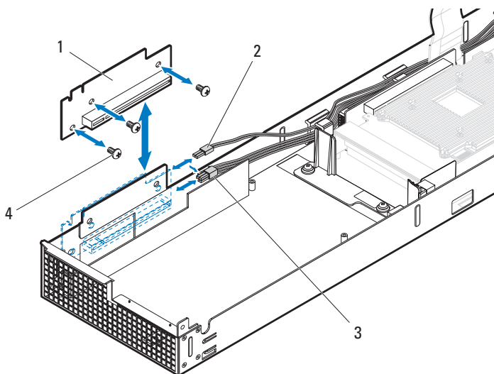
图 3-87. 卸下和安装正面 GPGPU 卡提升板
