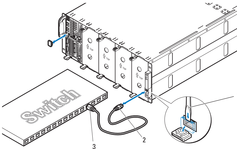
图 1-6. 非中央综合模式 — 以太网连接器
