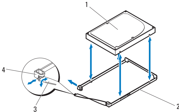
图 3-18. 从硬盘驱动器托盘中卸下硬盘驱动器，然后再安装
