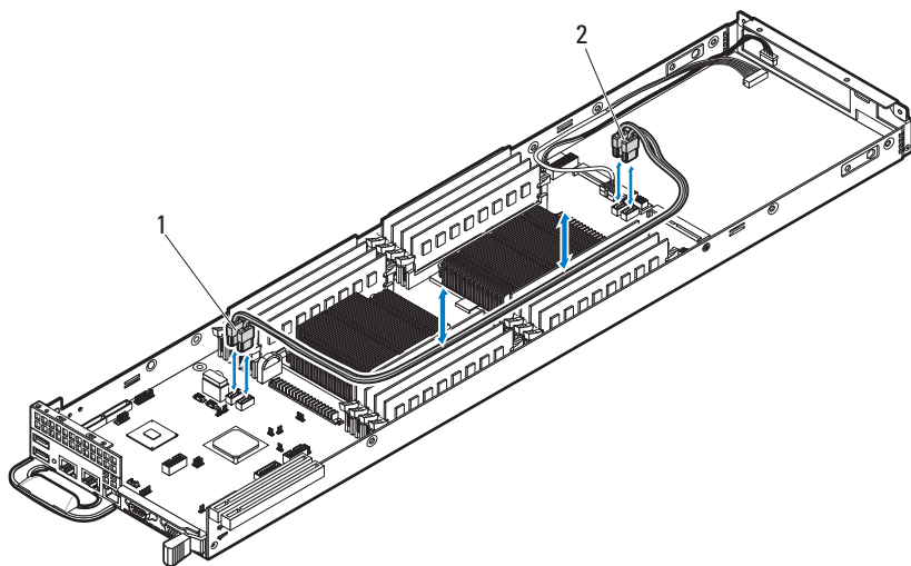
图 3-123. 卸下和安装 SATA 电缆
