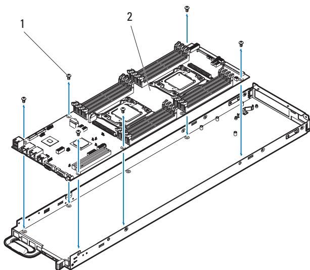
图 3-126. 卸下系统板
