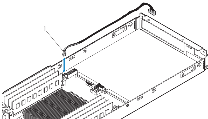
图 3-125. 卸下和安装 I2C 电缆
