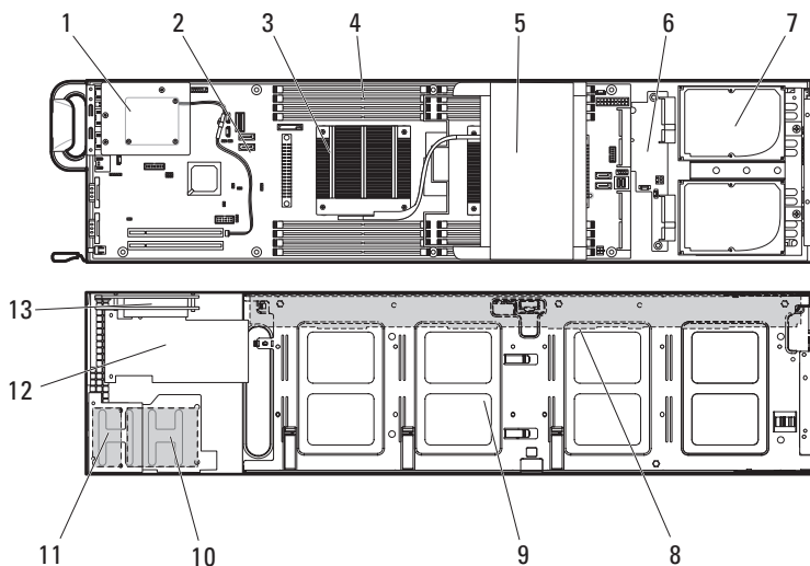
图 3-2. 带 2.5 英寸（8 驱动器托架）硬盘驱动器的 C8220X 的内部组件
