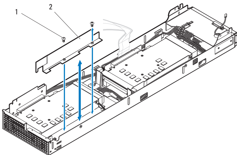
图 3-67. 卸下和安装空气导流板
