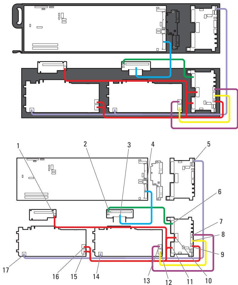
图 3-50. 正面和背面 NVIDIA Tesla M2090 GPGPU 卡部件的电缆布线
