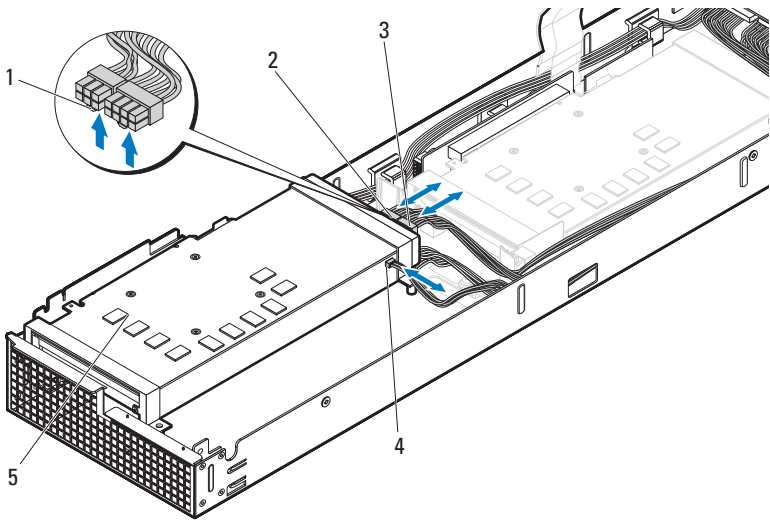
图 3-69. 卸下和安装正面 GPGPU 卡电缆
