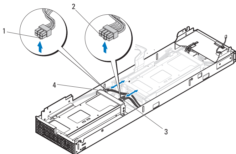
图 3-79. 卸下和安装正面 Xeon Phi 5110P/7120P 卡电缆
