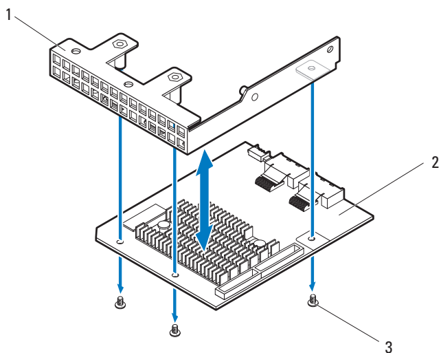
图 3-104. 卸下和安装 SAS 夹层卡
