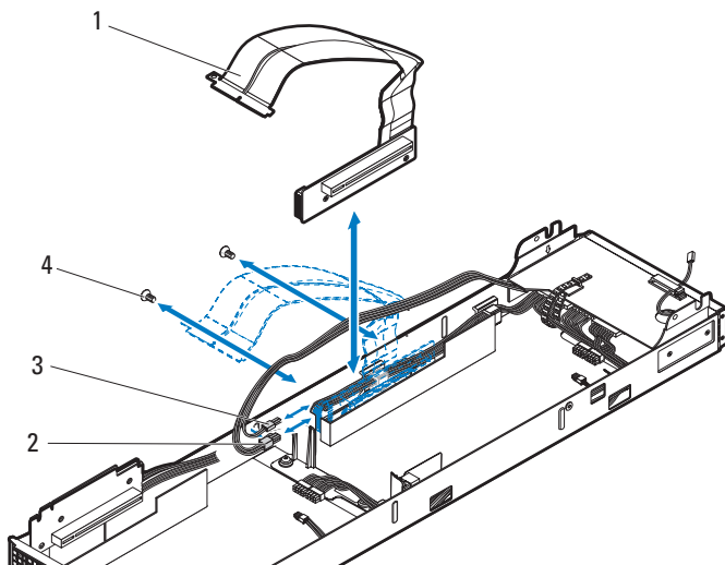
图 3-88. 卸下和安装背面 GPGPU 卡提升板
