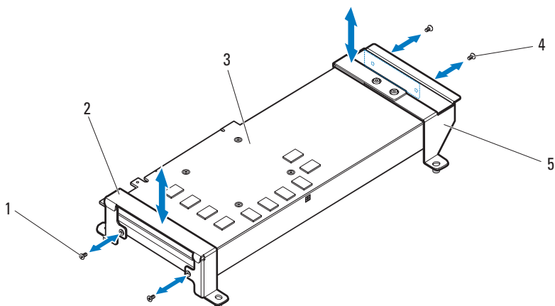
图 3-61. 卸下和安装正面 NVIDIA Tesla K10 GPGPU 卡
