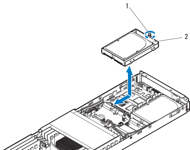
图 3-19. 卸下位于底座托架上的硬盘驱动器托盘，再将其安装
