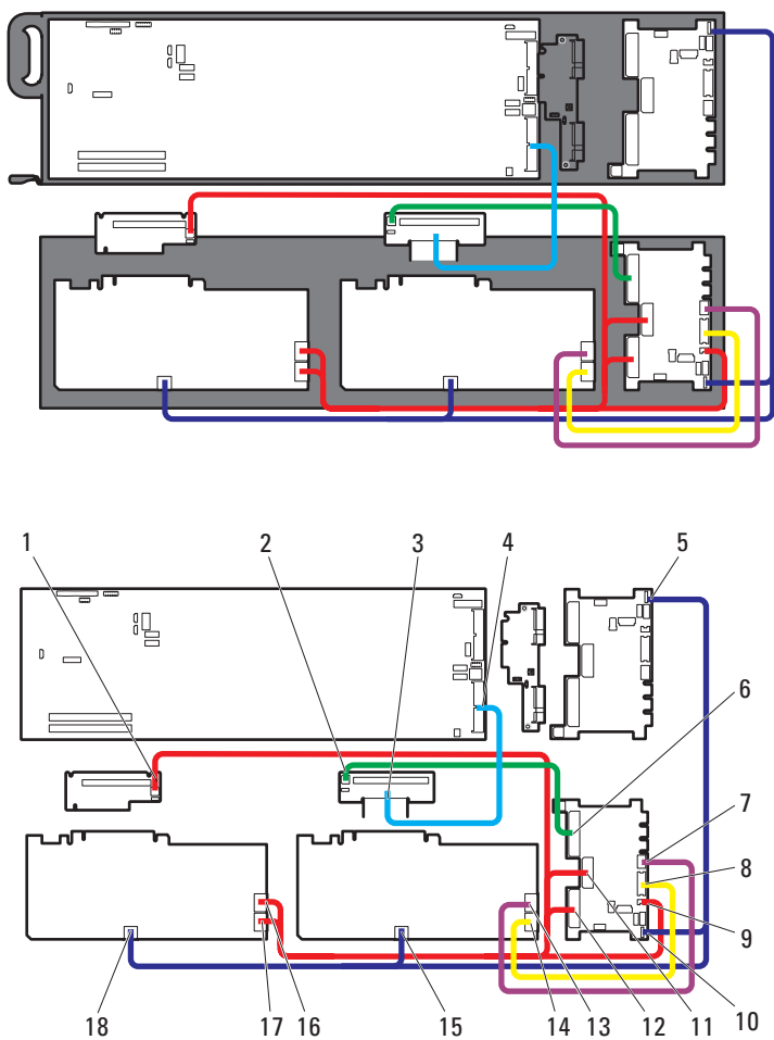
图 3-60. 正面和背面 NVIDIA Tesla K10 GPGPU 卡部件的电缆布线
