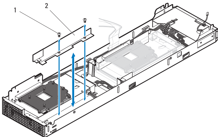
图 3-47. 卸下和安装空气导流板
