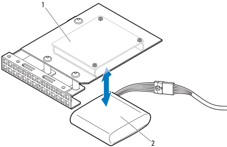
图 3-42. 卸下和安装 RAID 电池
