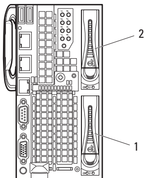
图 3-9. 前部访问的 2.5 英寸热插拔硬盘驱动器
