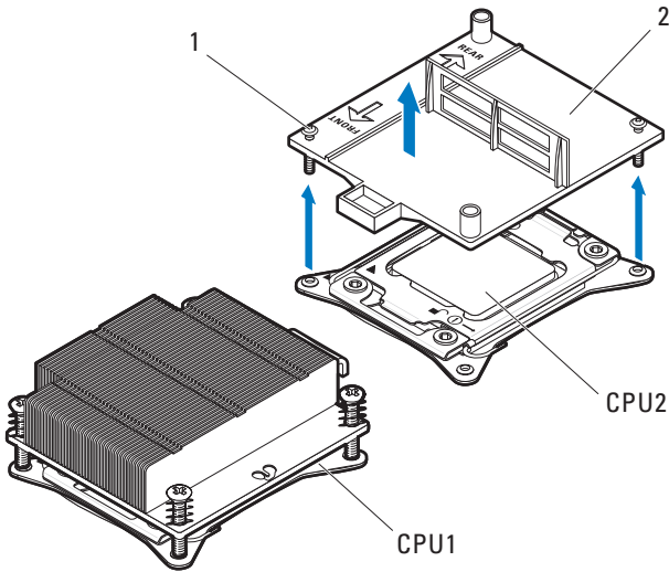
图 3-97. 卸下和安装散热器挡片
