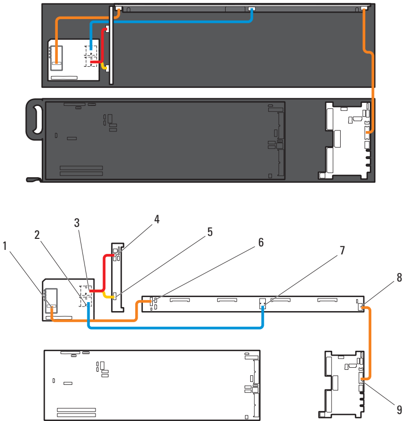
图 3-106. SAS 夹层卡的电缆布线 (3.5 英寸硬盘驱动器背板)
