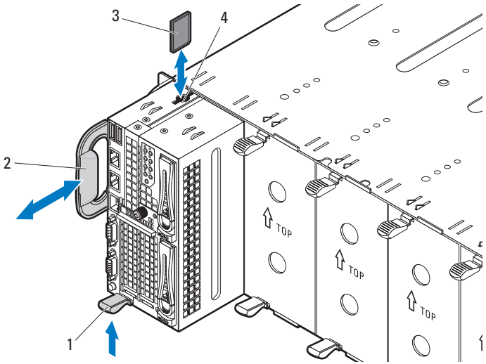
图 3-22. 卸下和安装 MicroSD 卡
