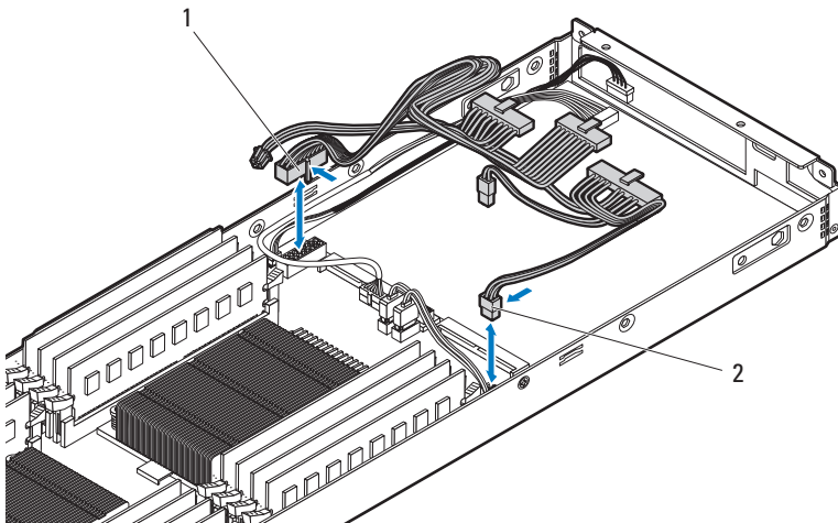
1,2 电源电缆
