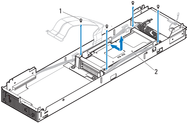
图 3-83. 卸下和安装背面 Xeon Phi 5110P/7120P 卡部件
