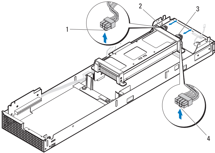
图 3-84. 卸下和安装背面 Xeon Phi 5110P/7120P 卡电缆
