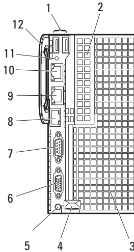
图 1-2. 底座功能部件 — 带 GPGPU/Xeon Phi 卡的 C8220X 双幅计算底座
