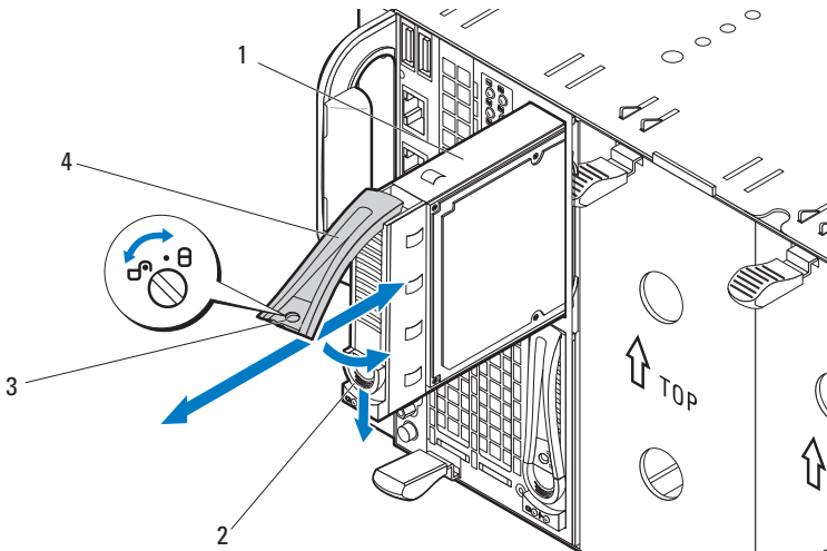
图 3-14. 卸下和安装硬盘驱动器托盘
