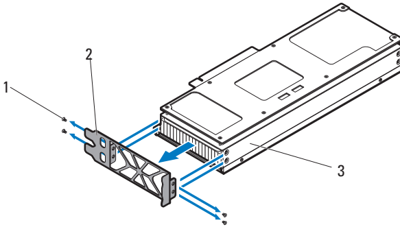
图 3-86. 卸下 Xeon Phi 5110P/7120P 卡支架
