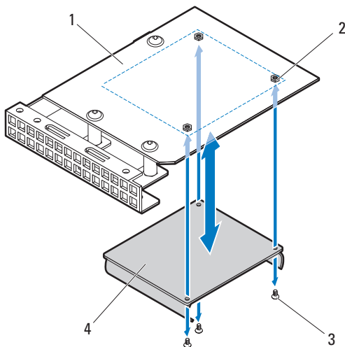
图 3-43. 卸下和安装电池座
