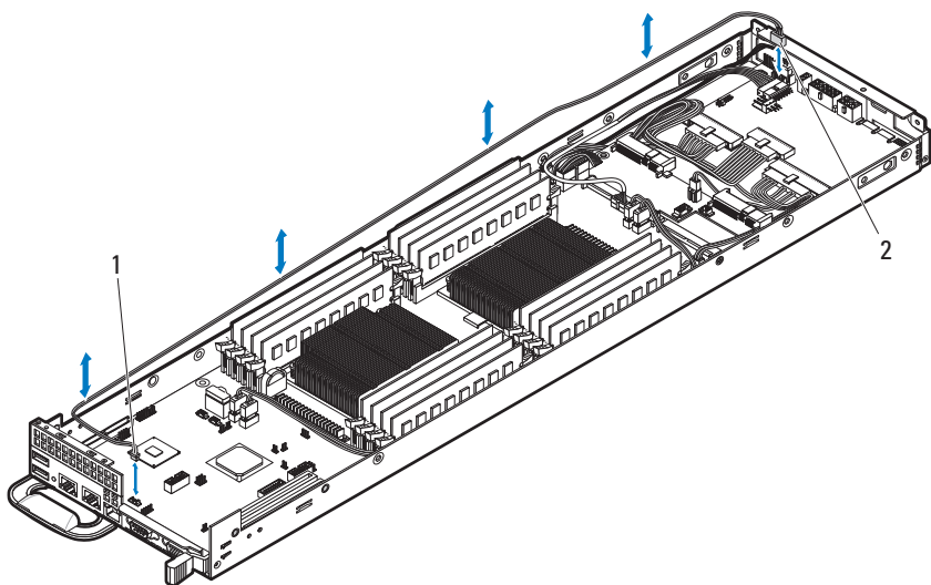
图 3-117. 拔下和安装 BMC 管理电缆
