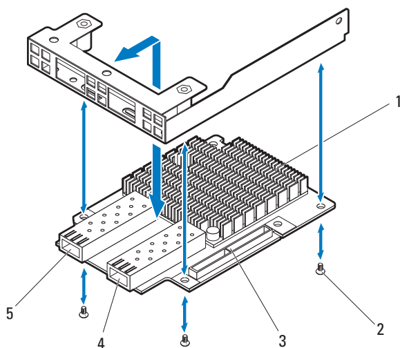
图 3-112. 卸下和安装 10 GbE 夹层卡
