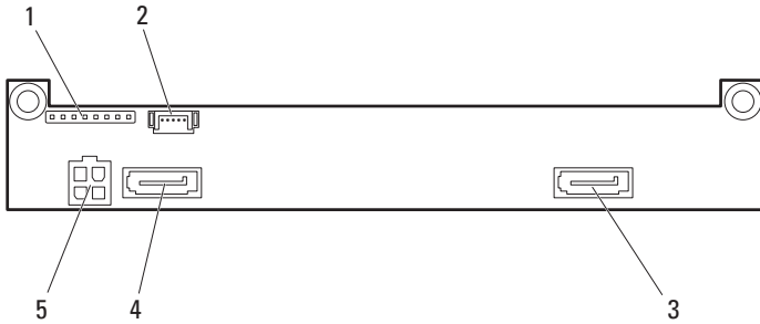
图 5-7. 2.5 英寸热插拔硬盘驱动器背板的正面视图
