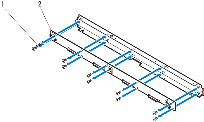
图 3-93. 卸下和安装 3.5 英寸硬盘驱动器固定框架背板
