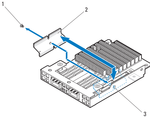
图 3-108. 卸下和安装夹层卡桥接板
