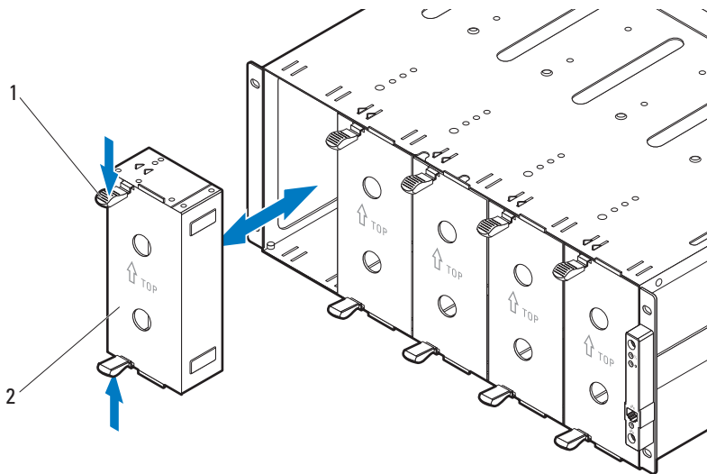
图 3-7. 卸下和安装双幅底座档片
