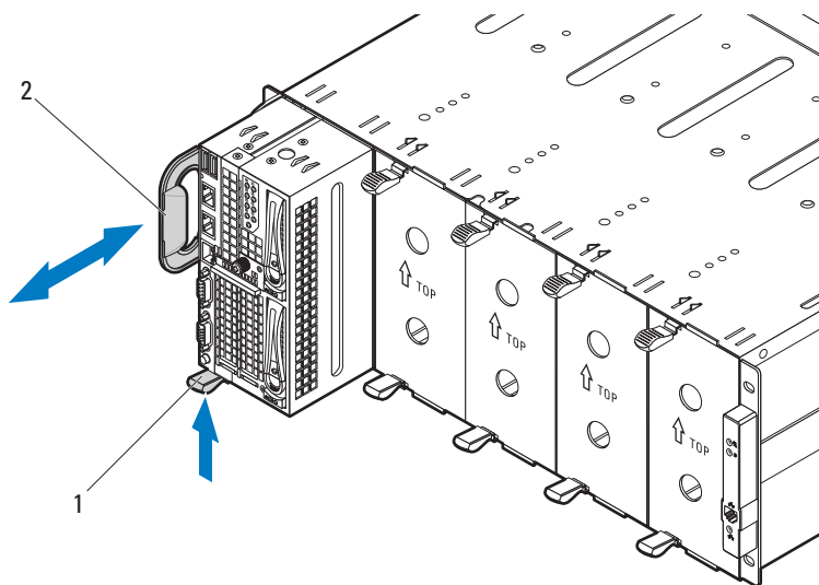
图 3-6. 卸下和安装底座
