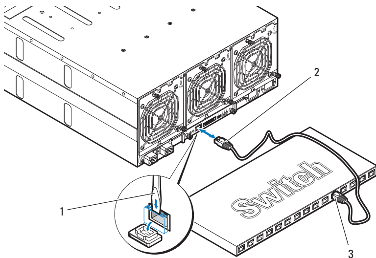
图 1-7. 非中央综合模式 — BMC 管理端口
